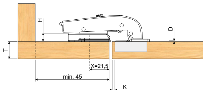
Nałożenie frontu zawias wpuszczany 90°
