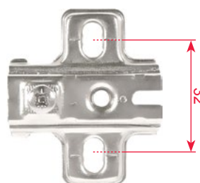
regulacja na fasoli
