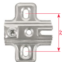
regulacja na fasoli
