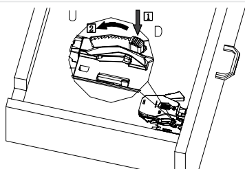
Regulacja wysokości
