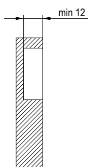
Wymiary montażowe puszek zawiasu i prowadnika
