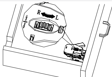
Regulacja boczna
