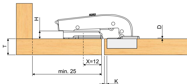
Nałożenie frontu zawias wpuszczany 90° z krótkim ramieniem
