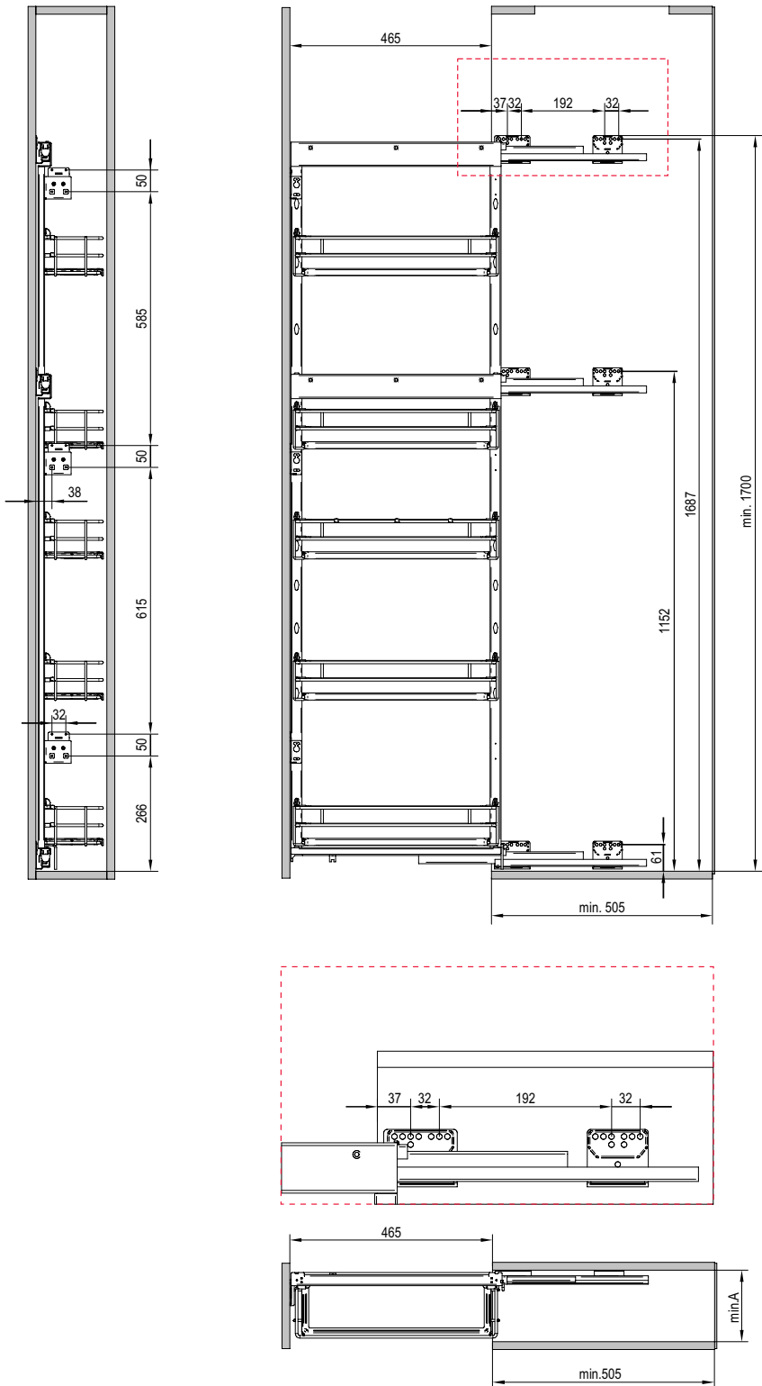
Montaż prowadnic do boku korpusu
