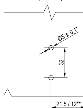
Wymiary montażowe puszek zawiasu i prowadnika
